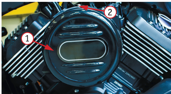
Фото 5.1 Воздушный фильтр: 1 – крышка, 2 – винты крепления
