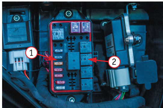
Фото 4.2 Отсек реле и предохранителей: 1 – предохранители, 2 – реле
