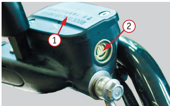
Фото 5.8 Уровень тормозной жидкости переднего тормоза: 1 –крышка; 2 – минимум
