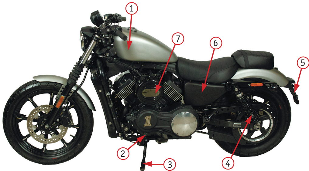
Фото 2.3. Вид слева: 1 – топливный бак; 2 – рычаг переключения передач; 3 – боковая подножка мотоцикла; 4 – задний амортизатор; 5 – крепление номерного знака; 6 – крышка аккумуляторного отсека; 7 – крышка воздушного фильтра
