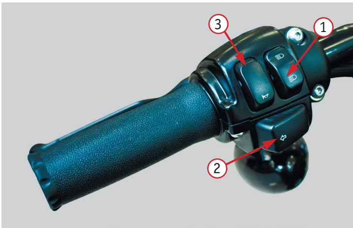
Фото 2.4 Левый комбинированный переключатель: 1 – кнопка переключения режима света фары (дальний свет/ближний свет); 2 – кнопка левого указателя поворота; 3 – кнопка звукового сигнала
