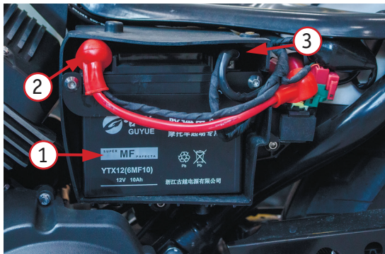
Фото 4.1 Аккумуляторный отсек: 1 – аккумуляторная батарея (АКБ); 2 – клемма «плюс»; 3 – клемма «минус»
