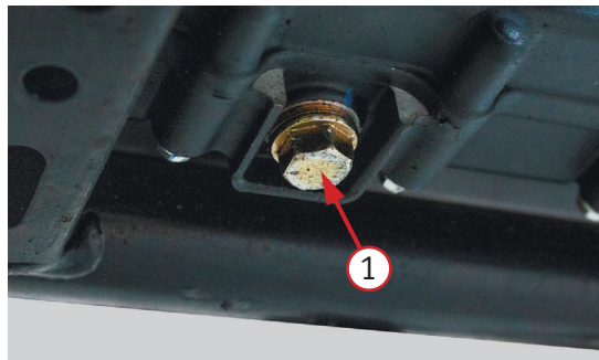
Фото 5.6. Болт слива масла - 1
