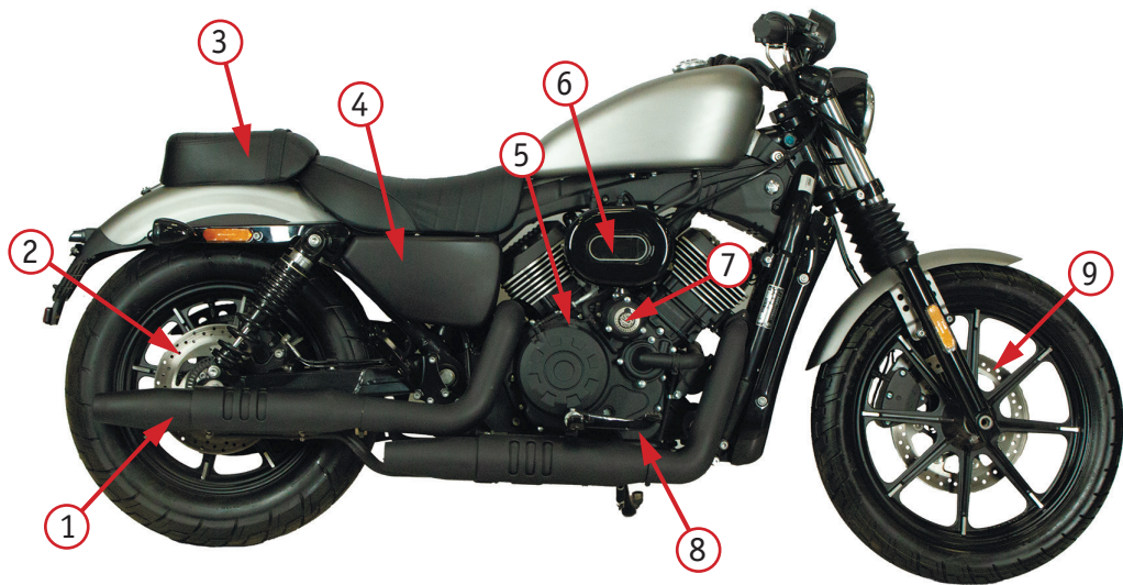
Фото 2.2. Вид справа: 1 – глушитель; 2 – задние дисковые тормоза; 3 – сиденье; 4 – крышка блока реле и предохранителей; 5 – заливная горловина для масла; 6 – защитная накладка бачка охлаждающей жидкости; 7 – масляный фильтр; 8 – педаль заднего тормоза; 9 – передние дисковые тормоза
