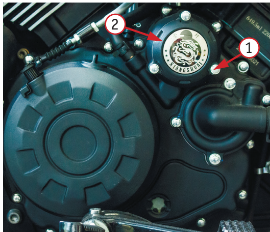
Фото 5.7. Замена масляного фильтра: 1 – винты крышки; 2 – крышка масляного фильтра
