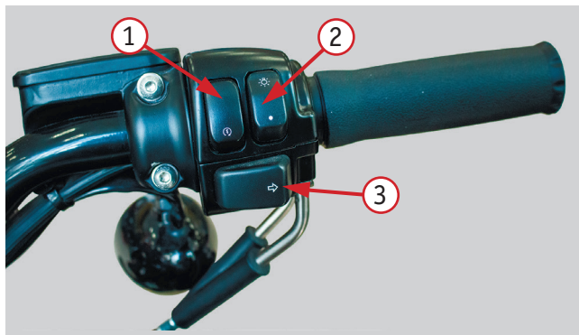
Фото 2.5. Правый комбинированный переключатель: 1 – кнопка электростартера; 2 – переключатель освещения; 3 – кнопка правого указателя поворота
