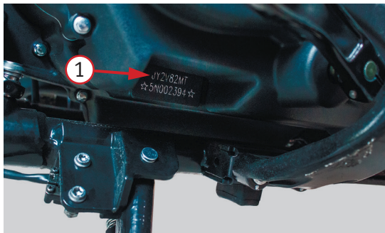
Фото 1.1. Слева на картере нанесен серийный номер двигателя – 1
