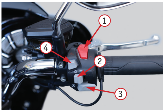
Фото 2.5. Правый комбинированный переключатель: 1 – переключатель включения/отключения питания; 2 – переключатель освещения; 3 – кнопка электростартера; 4 – кнопка аварийной сигнализации
