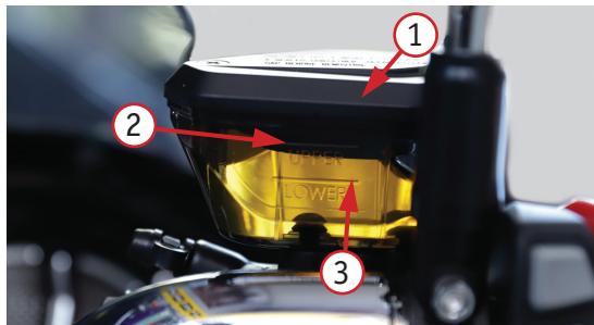
Фото 5.7.1 Уровень тормозной жидкости переднего тормоза: 1 – крышка; 2 – максимум; 3 – минимум
