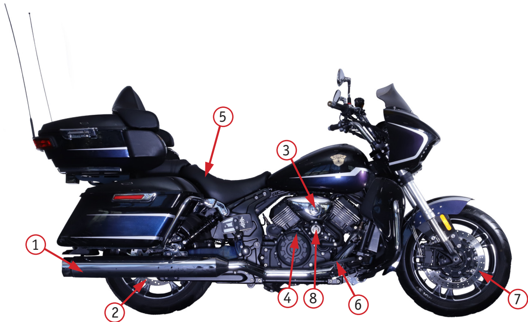
Фото 2.2. Вид справа: 1 – глушитель; 2 – задние дисковые тормоза; 3 – замок зажигания; 4 – заливная горловина для масла; 5 – сиденье; 6 – подножка водителя; 7 – передние дисковые тормоза; 8 – крышка масляного фильтра
